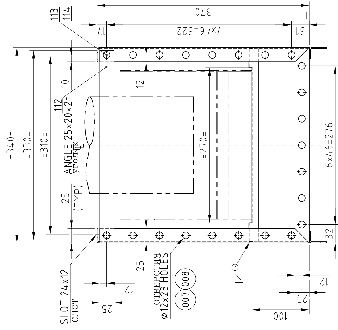
SECTION E-E СЕЧЕНИЕ
